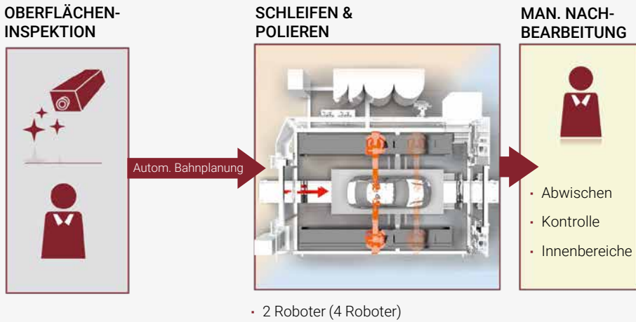
Abb. 36: Schleifen und Polieren in einer Zelle
