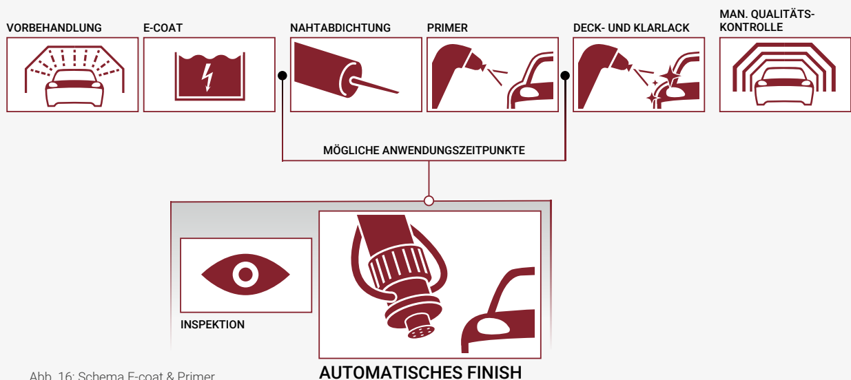
Abb. 16: Schema E-coat & Primer
