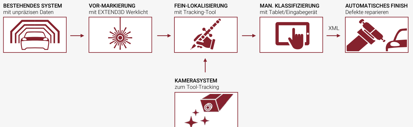
Abb. 14: Schema MDD Pro
