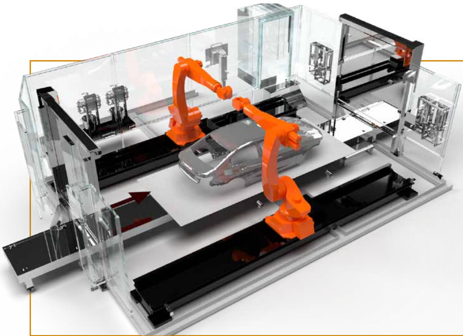
面漆和清漆施工后自动进行表面处理
