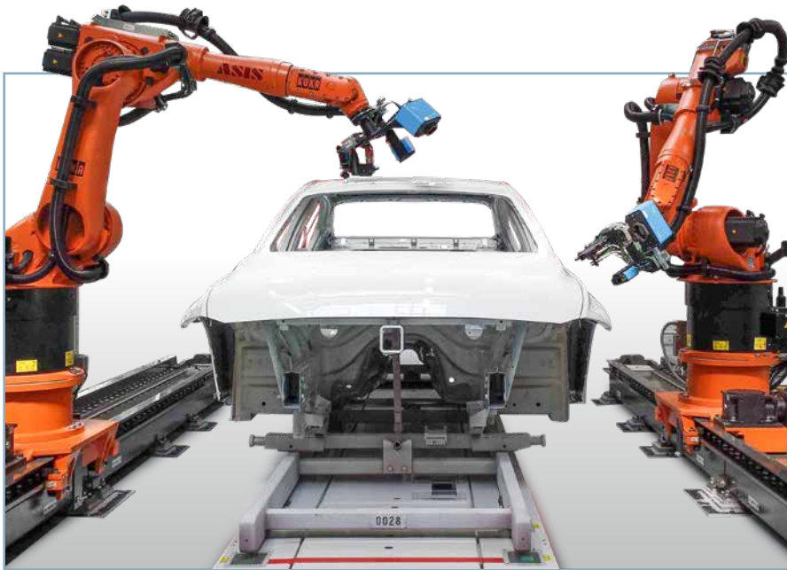
全自动的离线测量单元, 用于结构, 色调和涂层厚度的测量。
