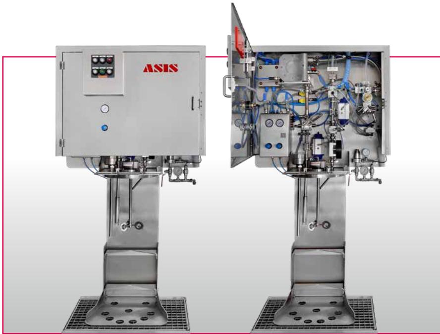
Das ASIS Special Color Supply System®: schneller Farbwechsel bei niedrigem Farbverlust für geringe Betriebskosten
